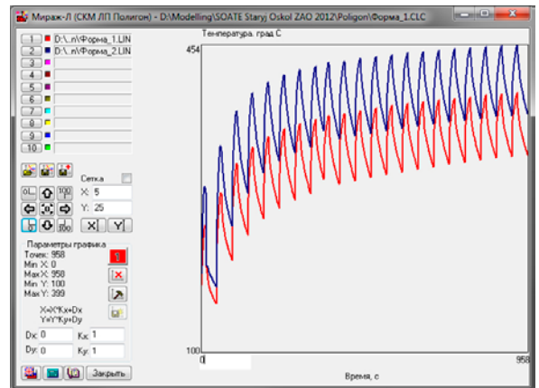
Контроль изменения температуры формы по циклам при ЛПД
