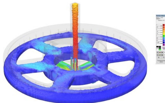
Литье в песчаную форму (ООО «КЗЭ "ДимАл"»)
